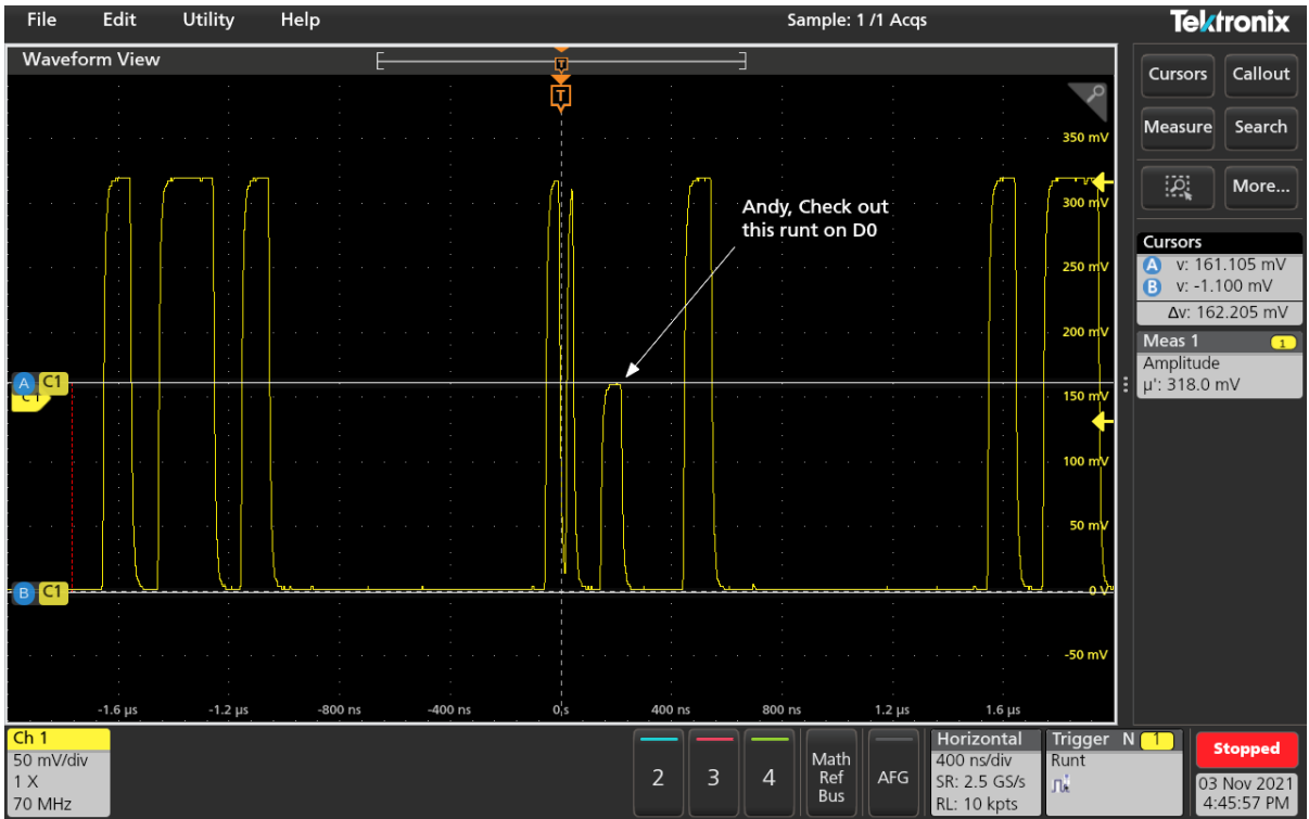
Beispiel für einen Impulsbreiten-Trigger, der zur Triggierung bei einem schmalen Impuls verwendet wird
