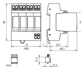
Maßbild DG MP TNS 275 FM
