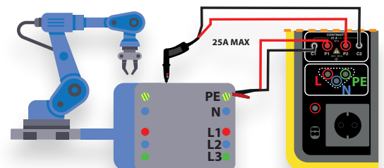
Hilfebildschirm bei der Durchgangsprüfung in Vierleitermessung bei 25 A (CA 6163)
