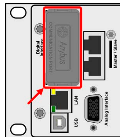
Bild 3 - Schnittstellenslot
