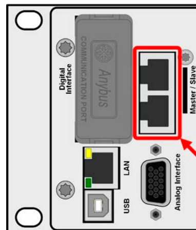
Bild 7 - Master-Slave-Busanschlüsse
