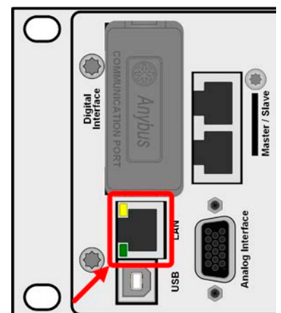
Bild 8 - LAN-Port
