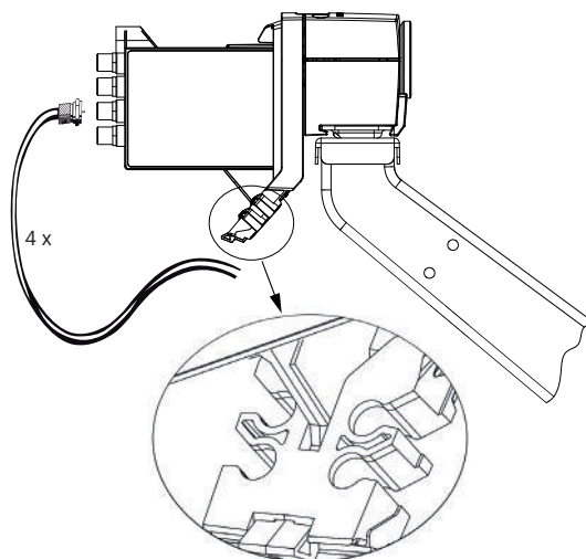
Abb. 5: Kabel montieren
