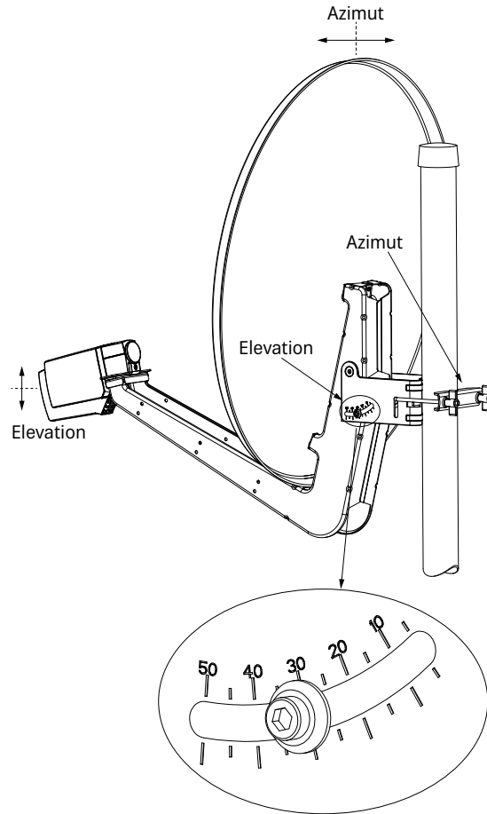
Abb. 6: Antenne ausrichten
