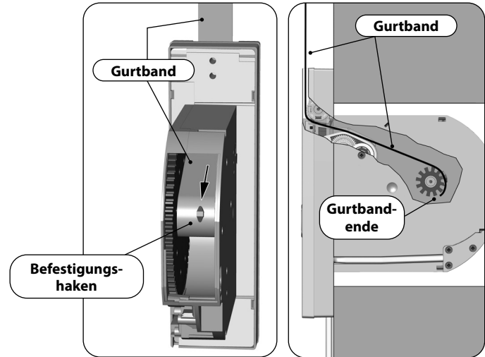
Gurtbandverlauf im Gurtwickler RolloTron premium
