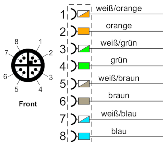
M12-Buchse
