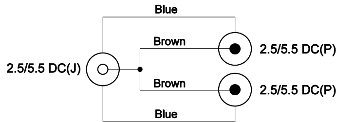
Wiring
