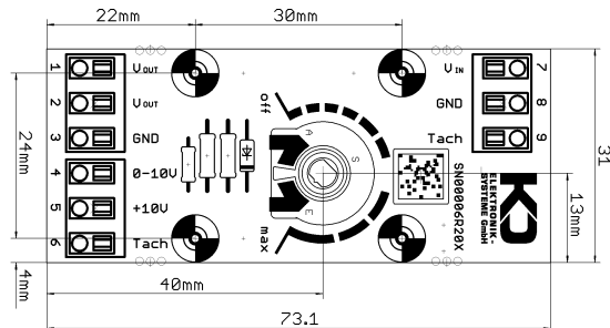
Abbildung 5 Ausführung ohne Gehäuse
