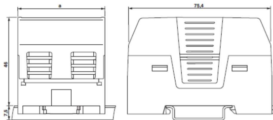
Abbildung 4 Ausführung im Gehäuse Breite a = 35,7 mm, ohne Achse gezeichnet
