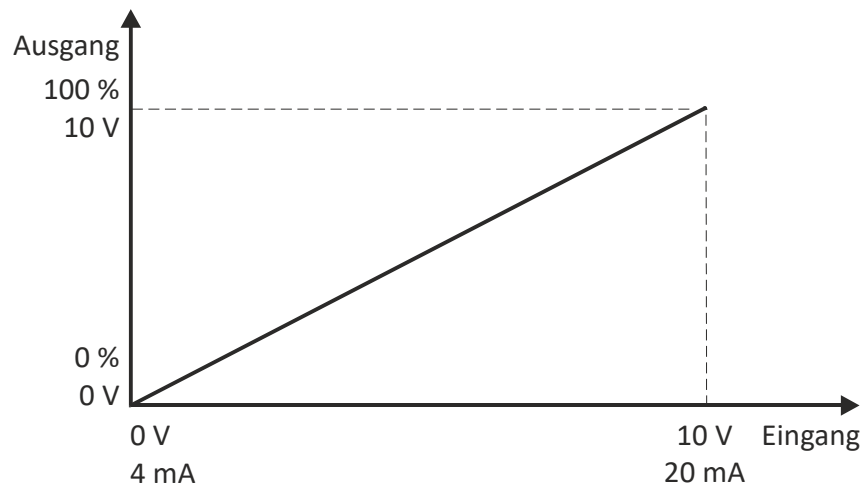
Abbildung 3 Kennlinie der Umsetzung der Eingangssignale auf die Ausgangssignale
