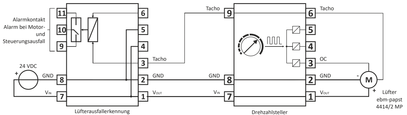
Abbildung 5 Anwendung des Drehzahlstellers zusammen mit einer Lüfterausfallerkennung der Fa. KD Elektroniksysteme
