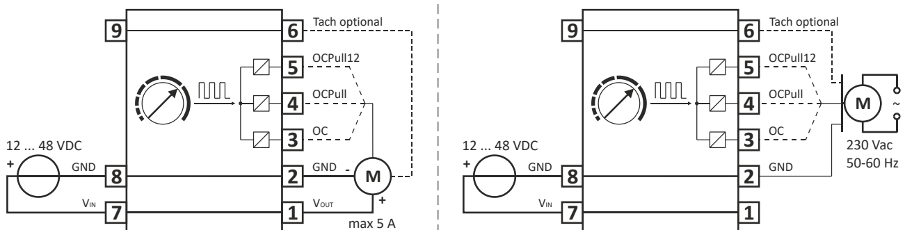
Abbildung 2 Typisches Anschluss-Schema für DC-Motoren (links) und AC-Motoren (rechts)
