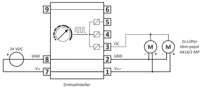
Abbildung 6 Anwendung als Drehzahlstellers für zwei ebm-papst Lüfter
