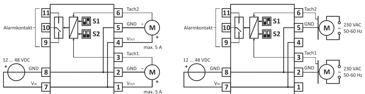
Abbildung 2 Typisches Anschluss-Schema für DC-Lüfter (links) und AC-Lüfter (rechts)
