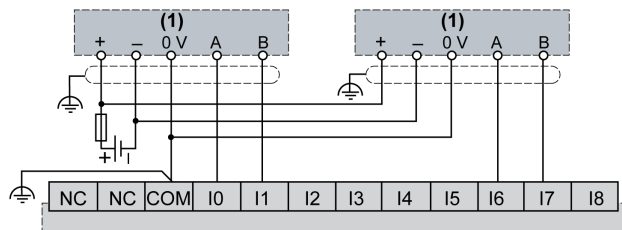
(1) Zweiphasengeber ohne Index
