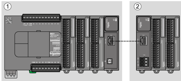
(1) Lokale Konfiguration (2) Dezentrale Konfiguration
