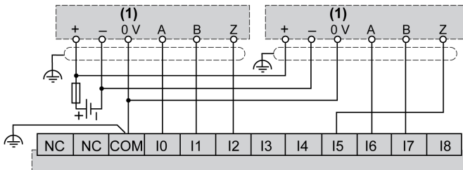
(1) Zweiphasengeber mit Index
