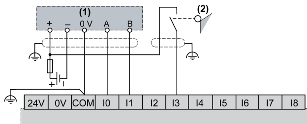
(1) Zweiphasengeber ohne Index
