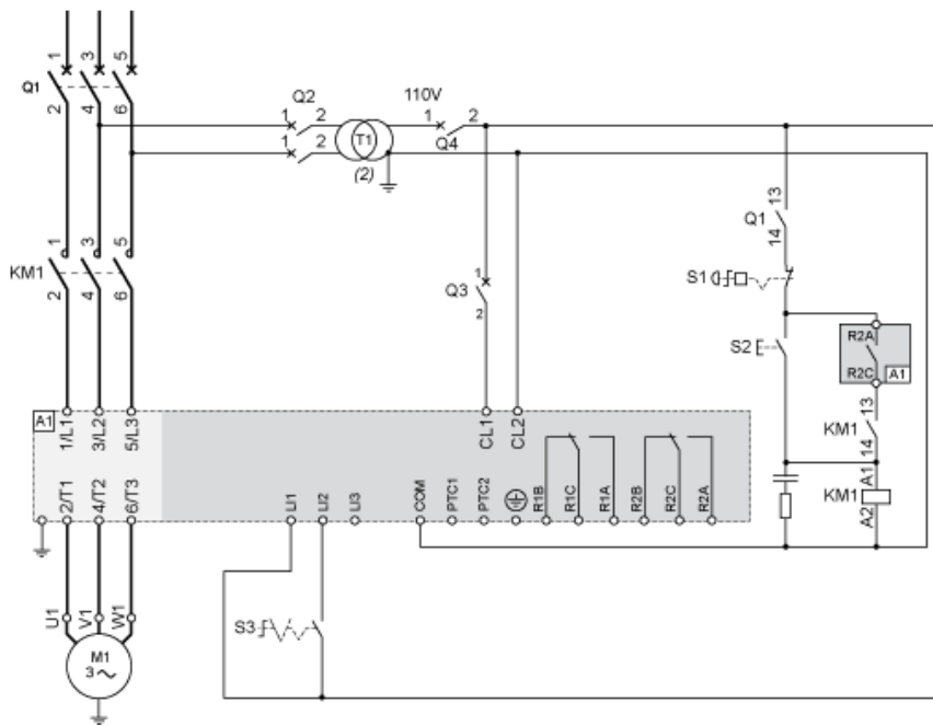
110-VAC-Steuerung, Logikeingänge (LI) 110 VAC, 2-Draht-Steuerung, freier Auslauf
