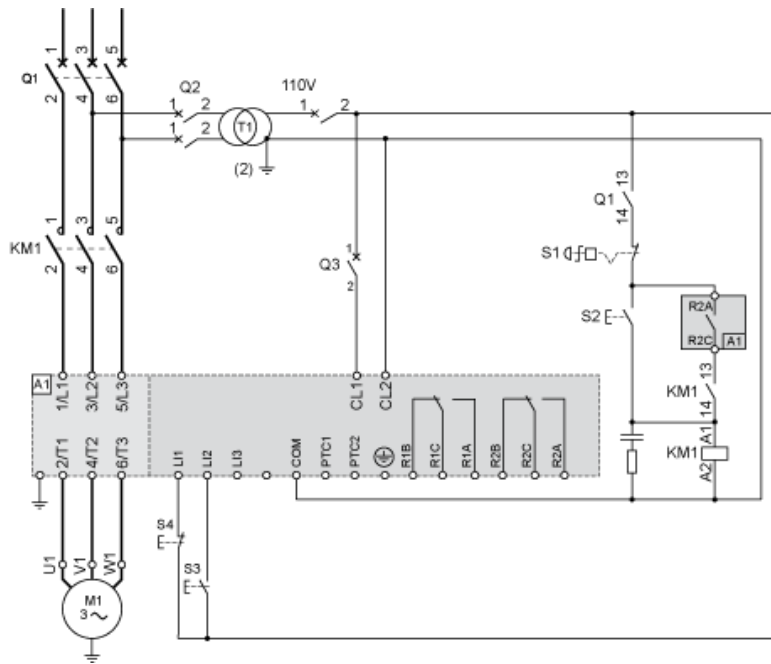
110-VAC-Steuerung, Logikeingänge (LI) 110 VAC, 2-Draht-Steuerung, freier Auslauf
