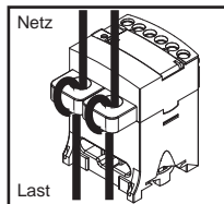
Verschleifungsoption (1 Schleife)
