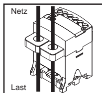
Durchgehende Verdrahtung
