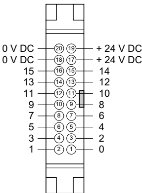
HE10 8 voies / Channels / Kanäle / canales / vie / vías
