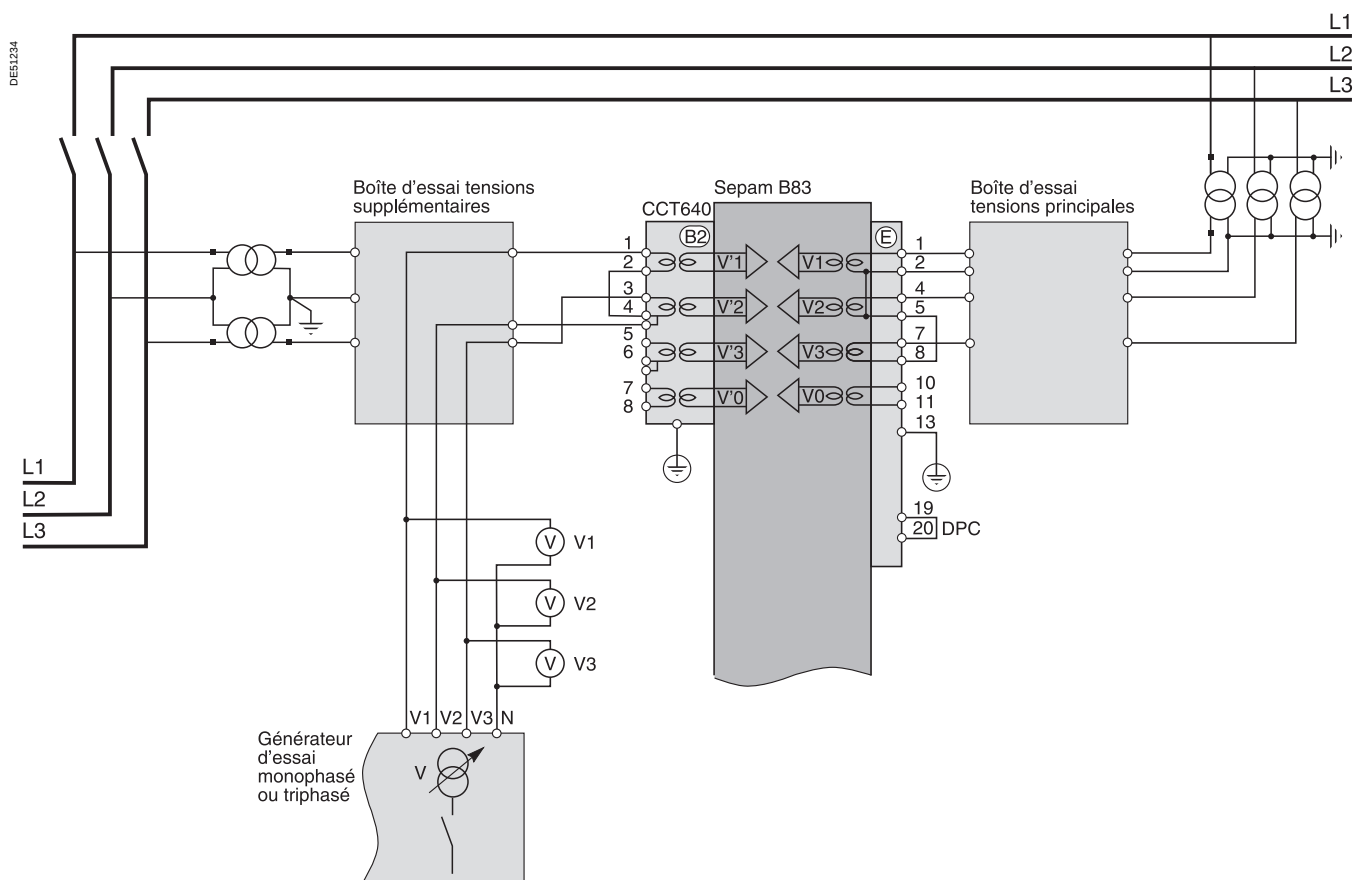
Schéma de principe avec 2 TP supplémentaires
