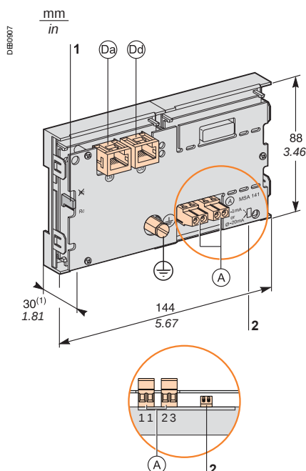
(1) 70 mm (2.8 in) avec câble CCA77x raccordé.
