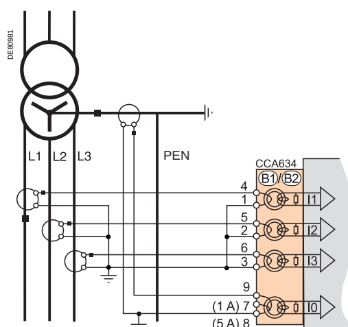
Raccordement sur réseau TN-C.
