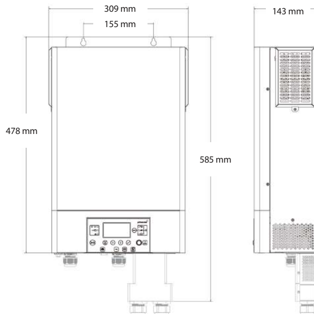
PSW-H-5KW-120/48V, PSW-H-6.5KW-120/48V and PSW-H-8KW-230/48V*
