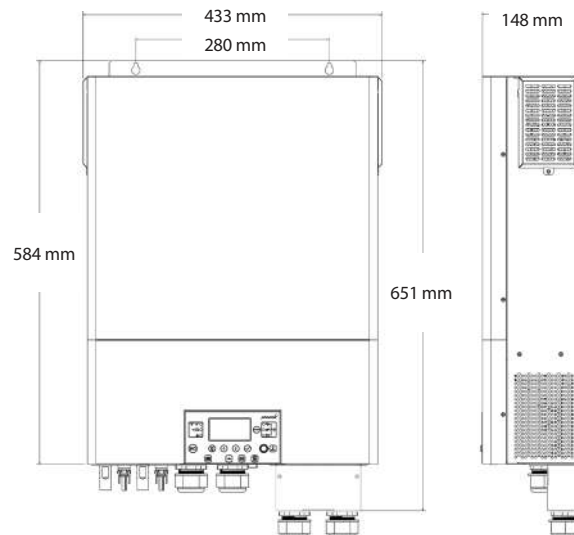
PSW-H-5KW-120/48V, PSW-H-6.5KW-120/48V and PSW-H-8KW-230/48V*
