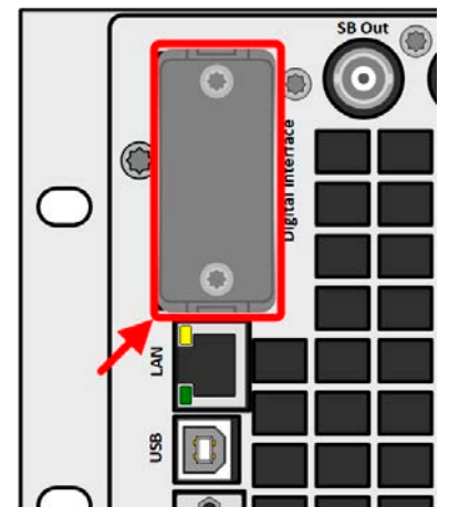
Bild 3 - Schnittstellenlot
