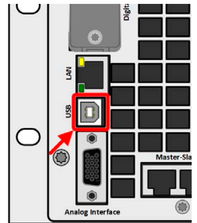
Bild 2- USB-Anschluß
