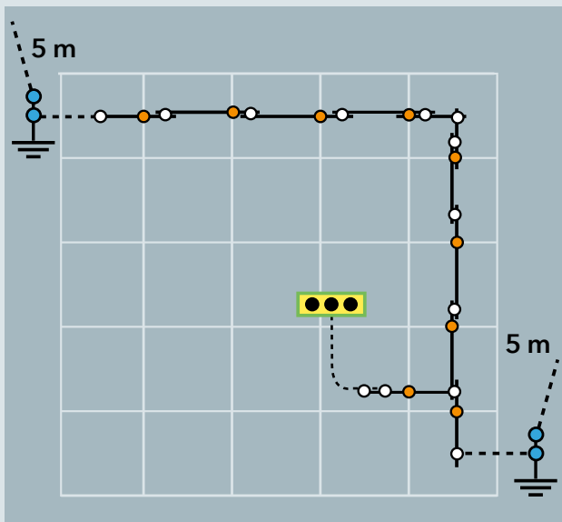
Variante 1.1: 1x Erdungsset Basis (2 x 5 m Tiefenerder inkl. 2 Anschlussfahnen)
