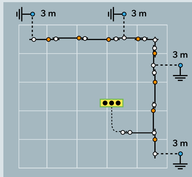
Variante 1.2: 1x Erdungsset Basis (4 x 3 m Tiefenerder)
