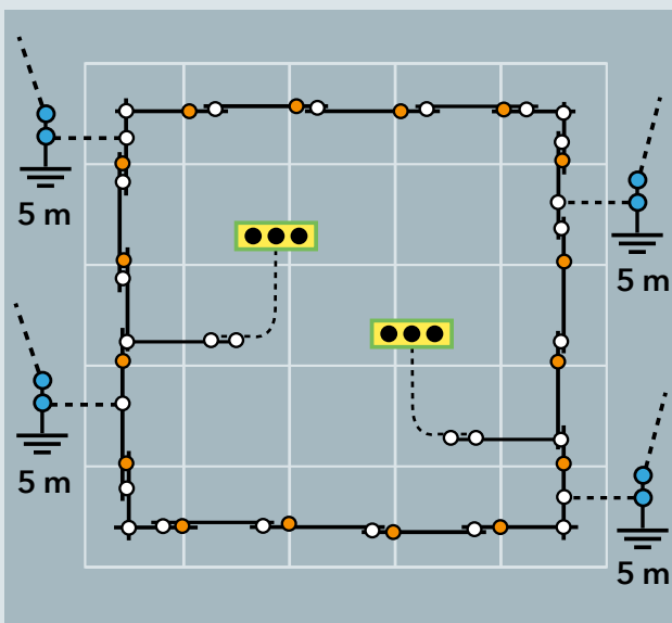
Variante 2: kombinierte Potentialausgleichsanlage (CBN) 2x Erdungsset Basis (4 x 5 m Tiefenerder inkl. 4 Anschlussfahnen)
