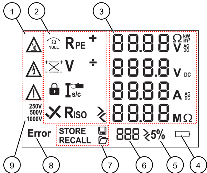
Abb. 2: Digitalanzeige
