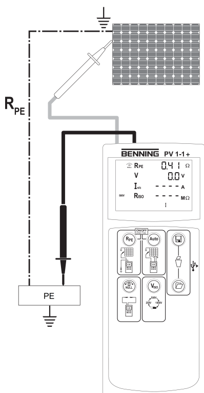
Abb. 4: Schutzleiterwiderstand
