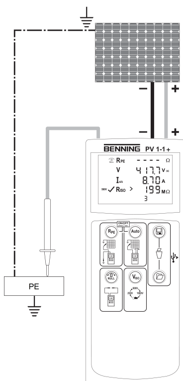
Abb. 5: Automatische PV-Messung
