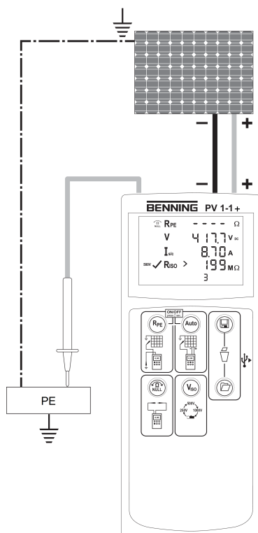
Abb. 8: Automatische PV-Messung
