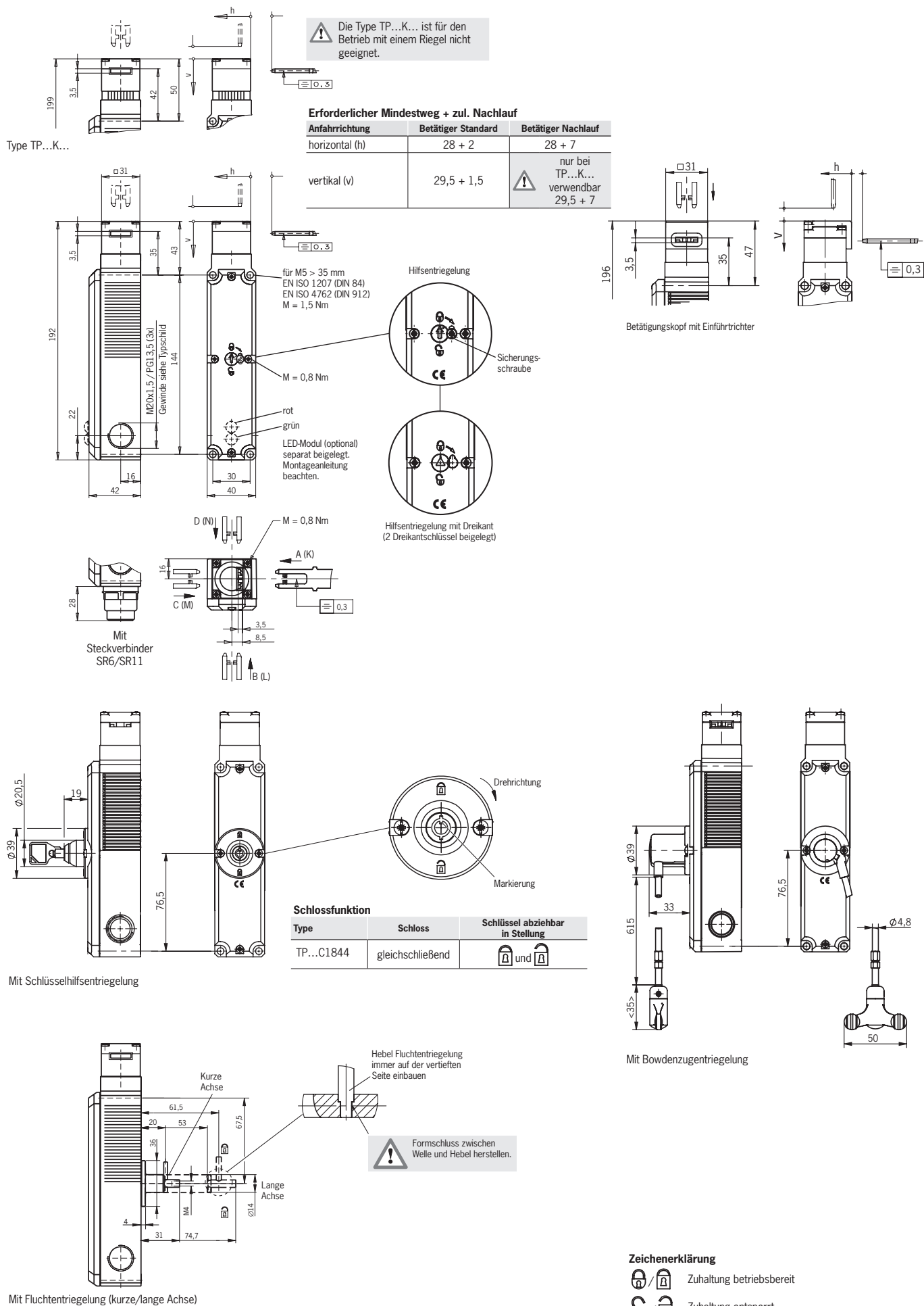
Bild 2: Maßzeichnung TP...
