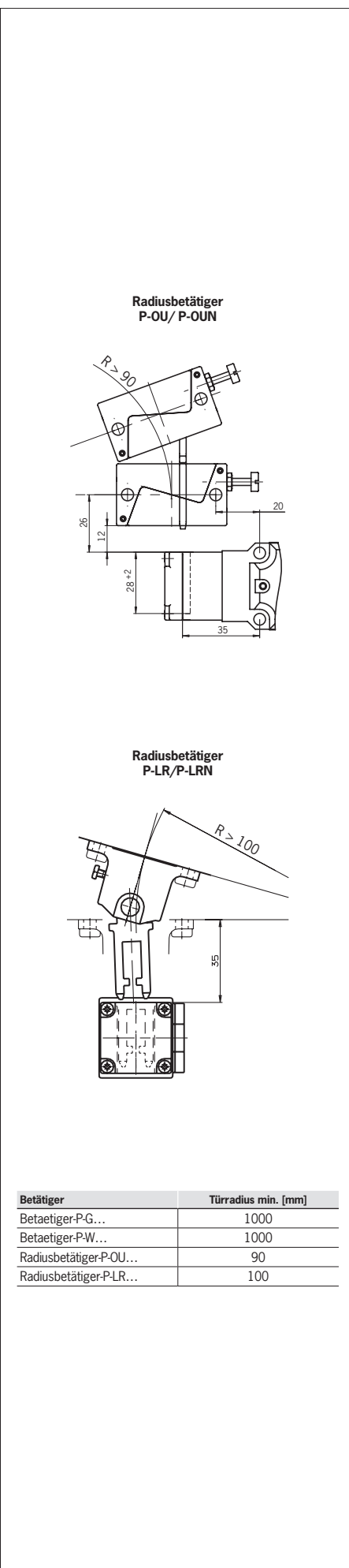
Bild 4: Minimale Türöffnungen
