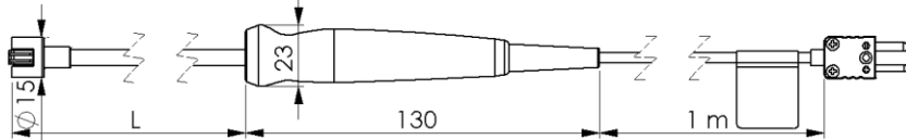
Oberflächenfühler mit Federbändchen Ø 15 mm
