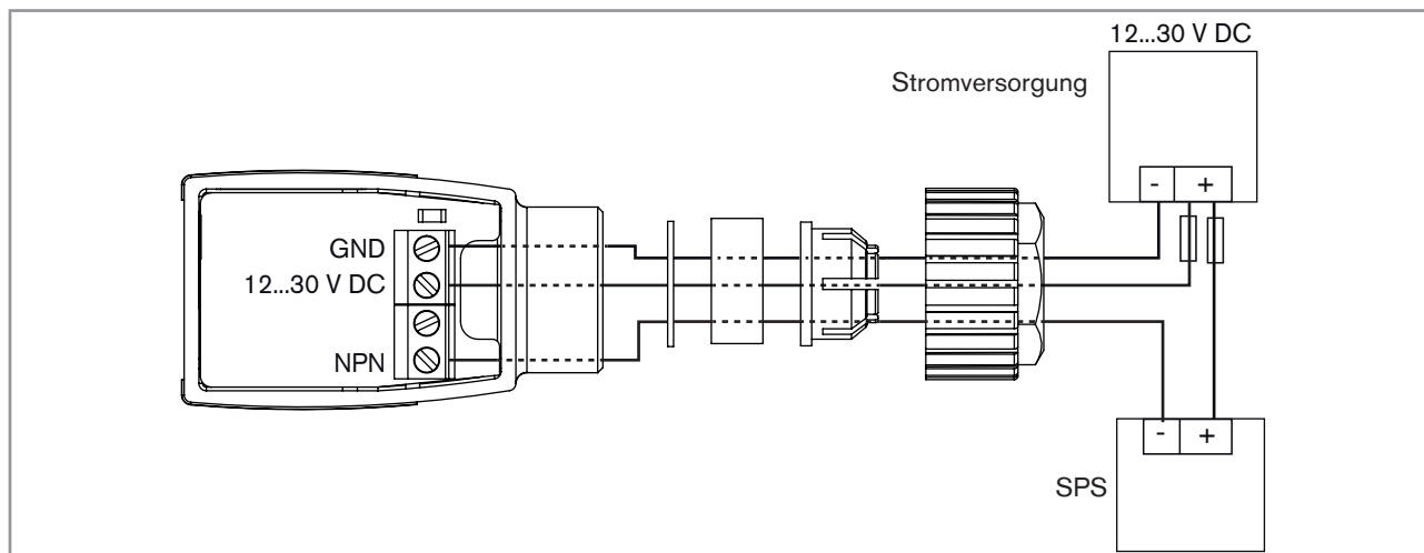
Bild 4: Gerät mit Kabelverschraubung – NPN-Anschluss des Transistorausgangs
