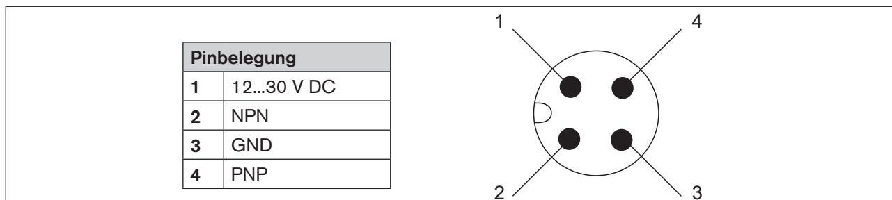
Bild 6: Pinbelegung des M12-Gerätesteckers (Ausführung mit 4-poligem M12-Gerätestecker)
