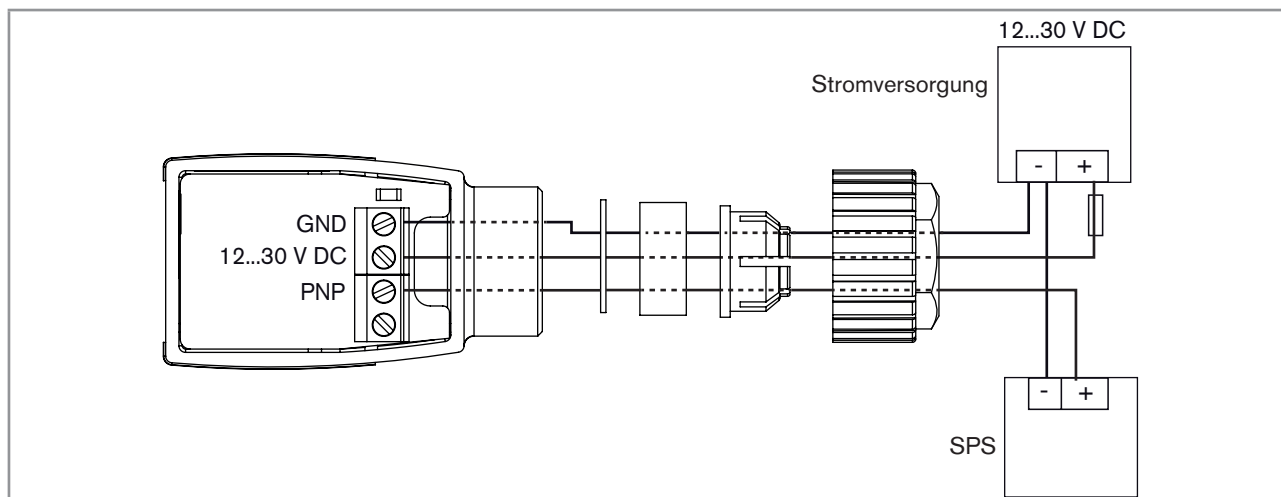
Bild 5: Gerät mit Kabelverschraubung – PNP-Anschluss des Transistorausgangs
