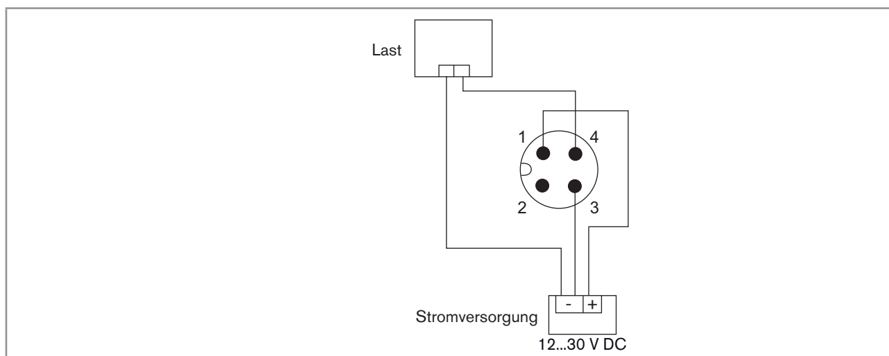
Bild 9: Gerät mit 4-poligem M12-Gerätestecker – PNP-Anschluss des Transistorausgangs
