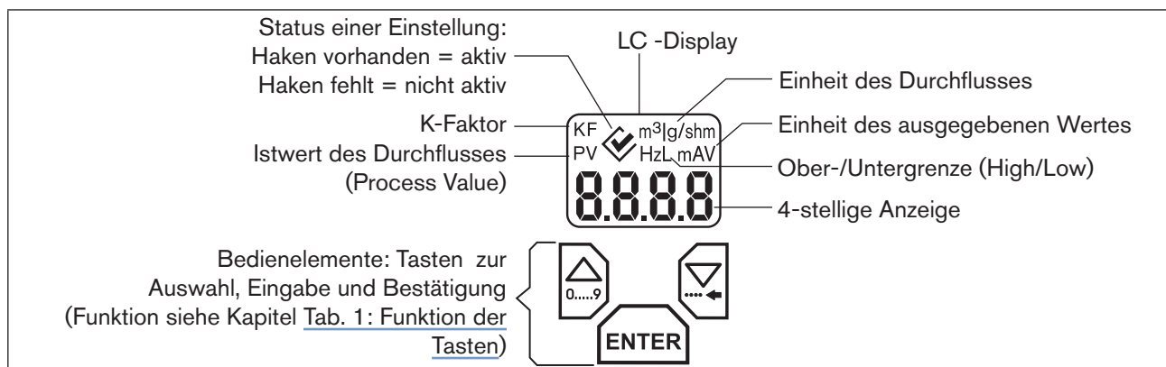
Bild 11: Displayeinheit
