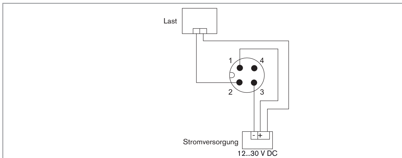
Bild 8: Gerät mit 4-poligem M12-Gerätestecker – NPN-Anschluss des Transistorausgangs
