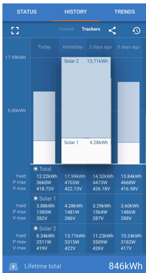
Abbildung 4. MPPT-Tracker- Ansicht
