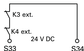
Abbildung 17: Automatische Aktivierung mit überwachter Kontakterweiterung K3/K4 - Zwangsgeführte Schütze
