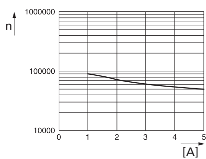
Abbildung 8: Schaltspielzahl AC-1
