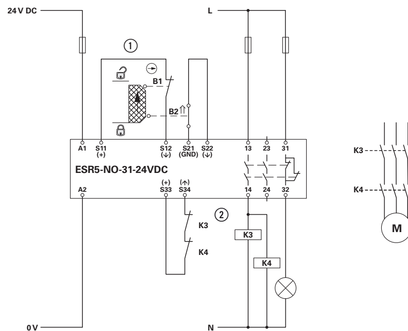
Abbildung 19: Zweikanalige Schutztür-Überwachung
