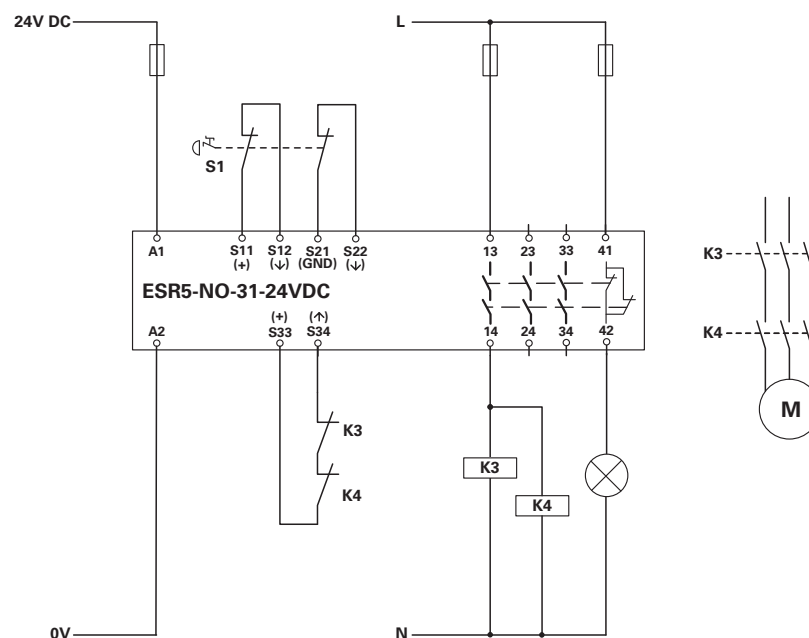
Abbildung 18: Zweikanalige Not-Halt-Überwachung
