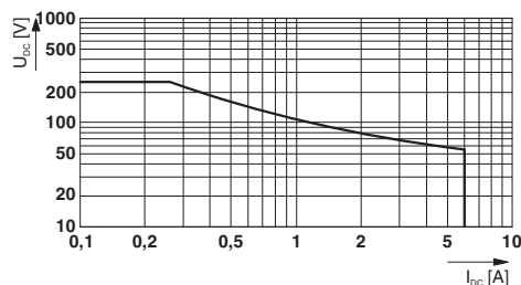
Abbildung 7: Lastkurve des Relais – Ohmsche Last
