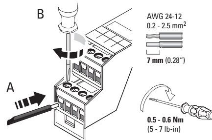
Abbildung 13: Anschluss der Leitungen
