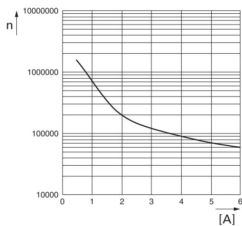
Abbildung 8: Schaltspielzahl AC-1
