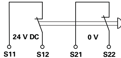
Abbildung 14: Zweikanaliger Anschluss mit Querschlusserkennung
