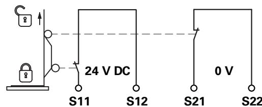
Abbildung 15: Zweikanalige Schutztür-Schaltung, zwei Öffnerkontakte
