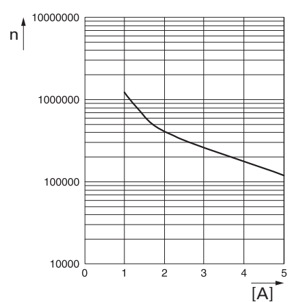
Abbildung 11: Schaltspielzahl DC-13
