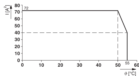
Abbildung 4: Derating-Kurve – horizontale Einbaulage, ohne Abstand
