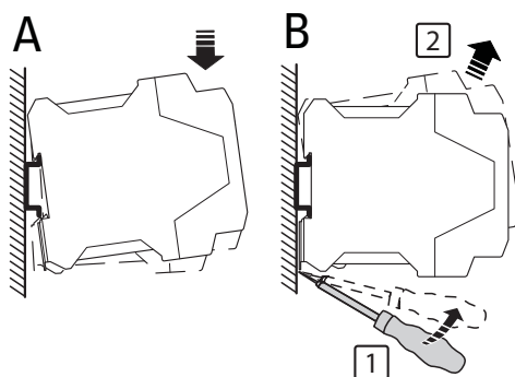
Abbildung 12: Montage A und Demontage B
