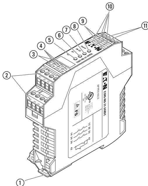
Abbildung 1: ESR5-NO-31-24VDC
