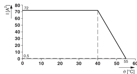
Abbildung 5: Derating-Kurve – vertikale Einbaulage, ohne Abstand
