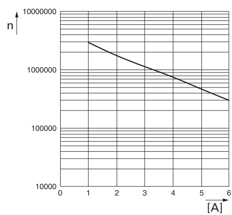
Abbildung 9: Schaltspielzahl DC-1
