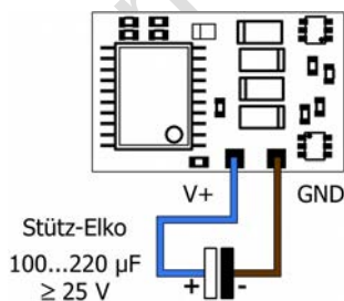
Anschluss eines Stütz-Kondensators ("Puffer-Elkos")
