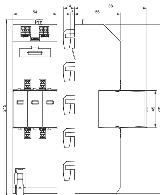
Typ 7P.04.8.255.Zxxx
