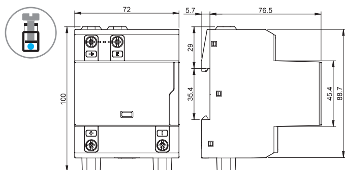
Typ 7P.13.9.000.x006 Schraubklemmen
