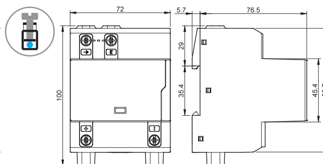
Typ 7P.13.9.500.x006 Schraubklemmen
