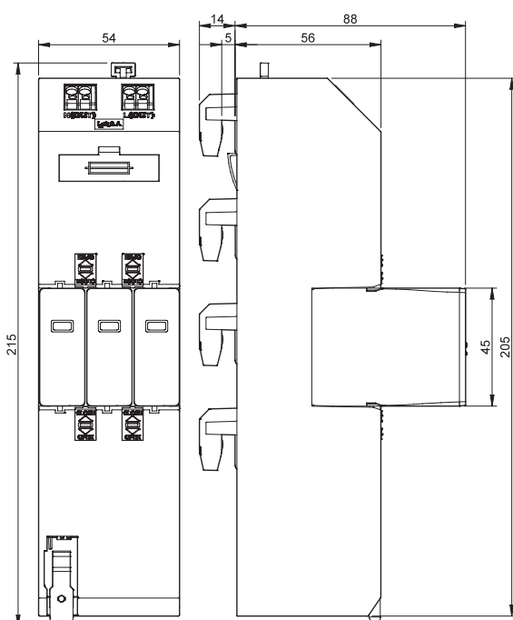
Typ 7P.03.8.255.Zxxx
