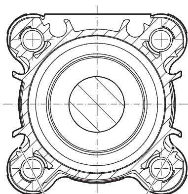
Typ: Zylinder mit Profilrohr ø 32 ... 125 mm
