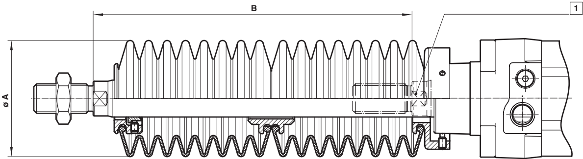
1 Kolbenstange ohne Faltenbalg
