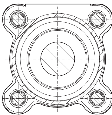
Typ: Zylinder mit Rundrohr ø 32 ... 125 mm
