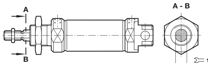
1 Dämpfungsschraube
