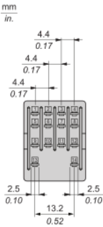
Stecker-Seitenansicht
