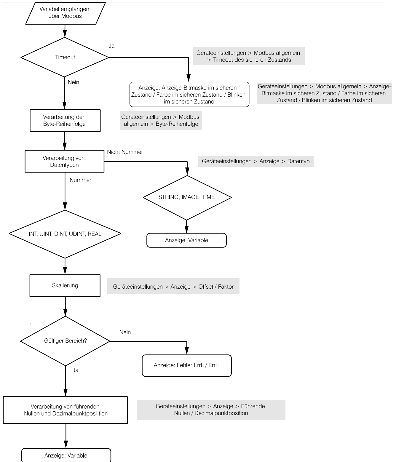
Abb. 4.1 Anzeige-Betriebsflussdiagramm
