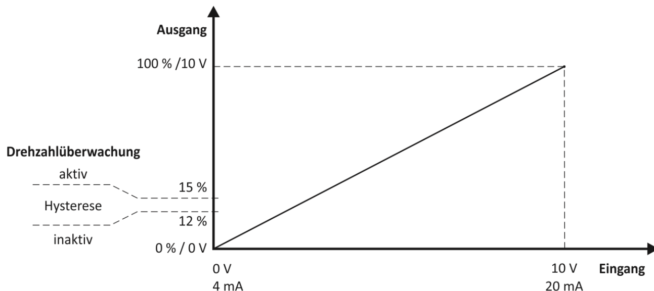
Abbildung 3 Umsetzung der Eingangssignale auf das Drehzahl-Steuersignal und Abhängigkeit der Drehzahlüberwachung
