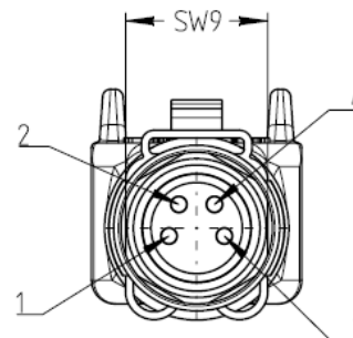
Maß- / Schemazeichnung
