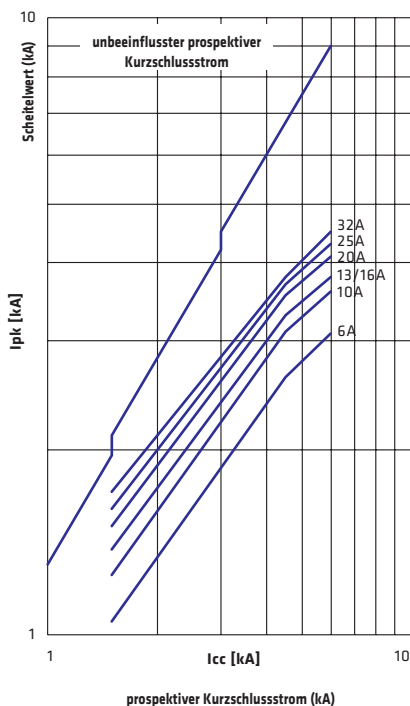
MDC - 3P, 4P - 400V Versionen
