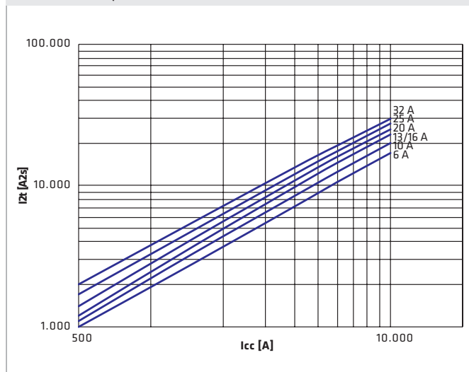
MDC 60 - 1P+N, 2P - 230V Versionen
