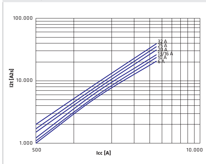
MDC 45 - 3P, 4P - 230/400V Versionen
