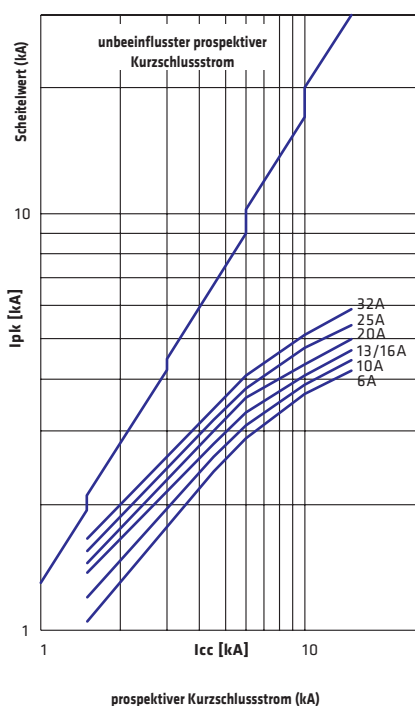
MDC - 1P+N, 2P - 230V Versionen
