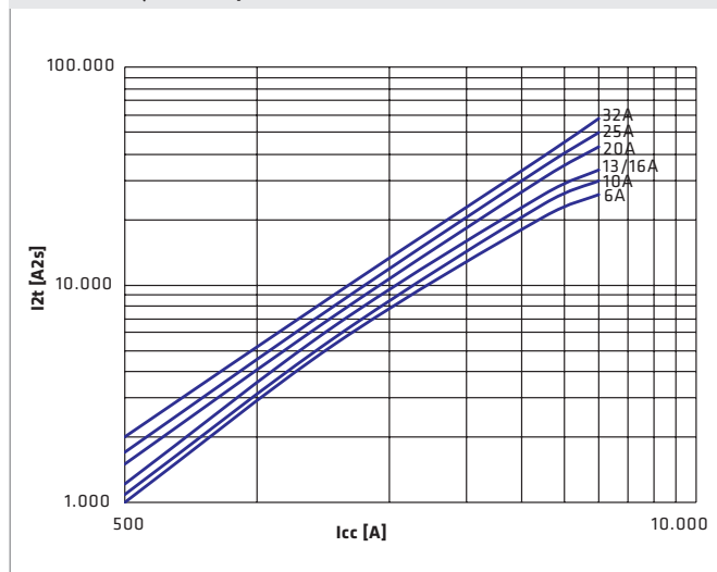
MDC 60 - 3P, 4P - 230/400V Versionen
