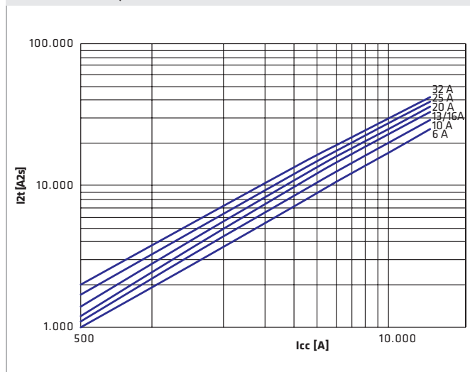
MDC 100 - 1P+N, 2P - 230V Versionen
