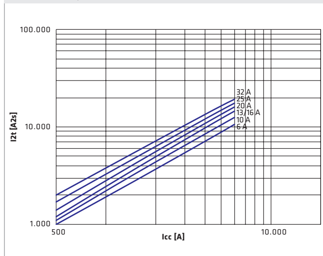
MDC 45 - 1P+N, 2P - 230V Versionen
