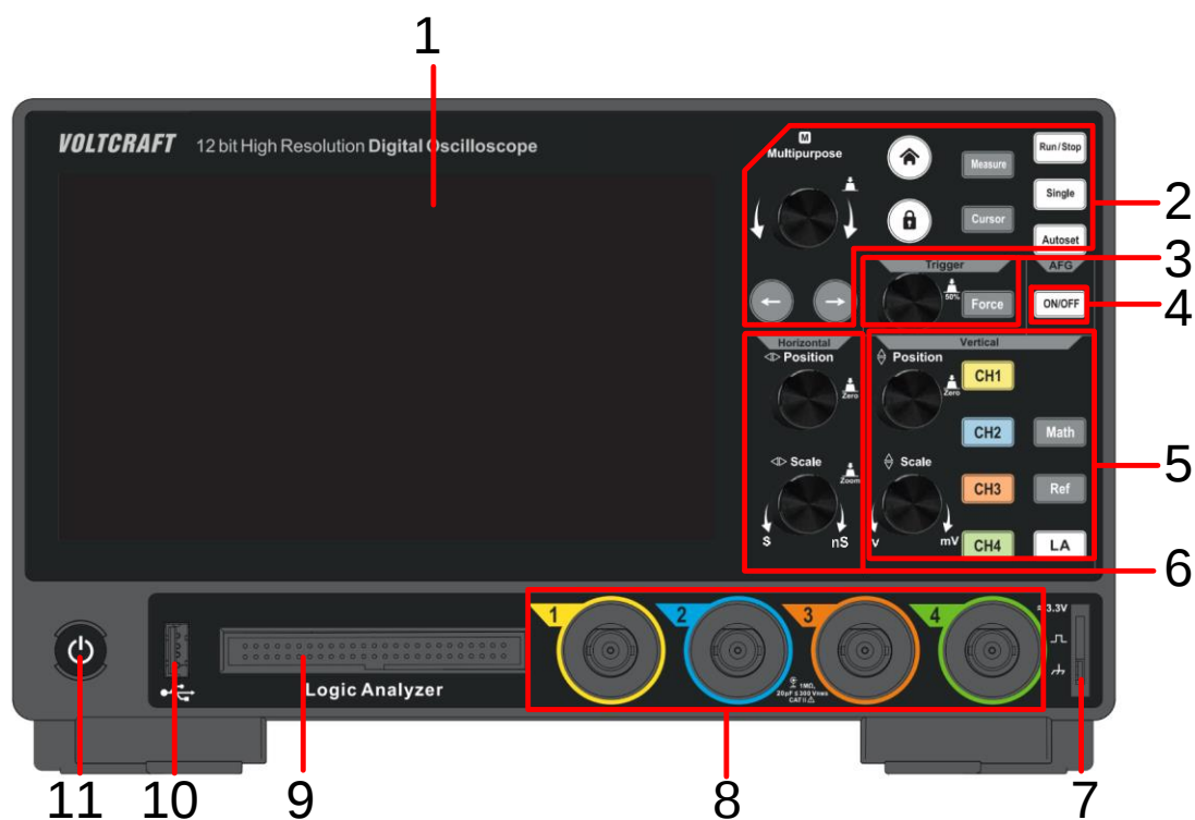
Abbildung 3-1: Vorderseite
