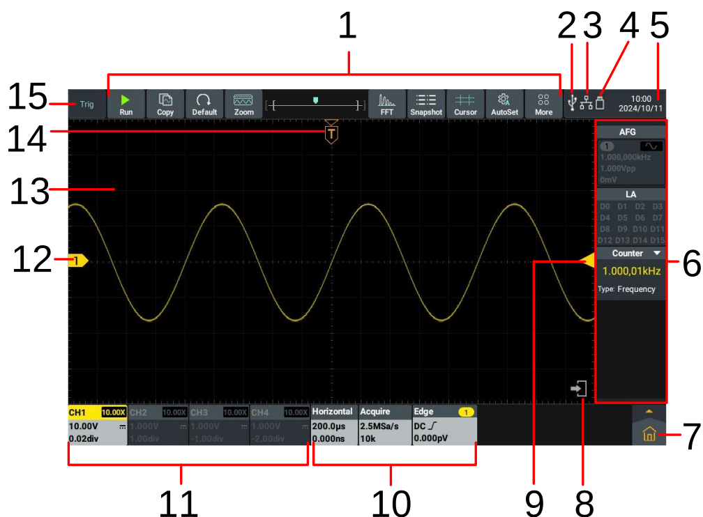
Abbildung 3-3: Benutzeroberfläche
