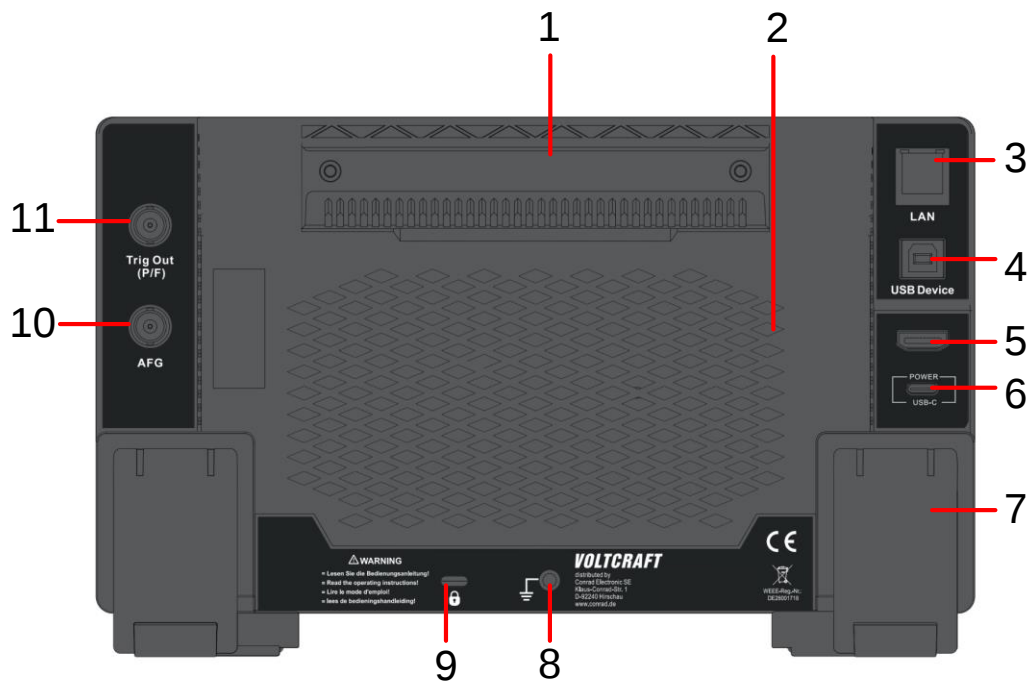
Abbildung 3-2: Rückseite
