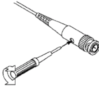
Abbildung 3-6: Prüfspitze einstellen
