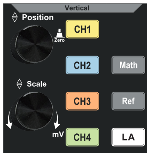
Abbildung 5-4: Vertikaler Steuerungsbereich
