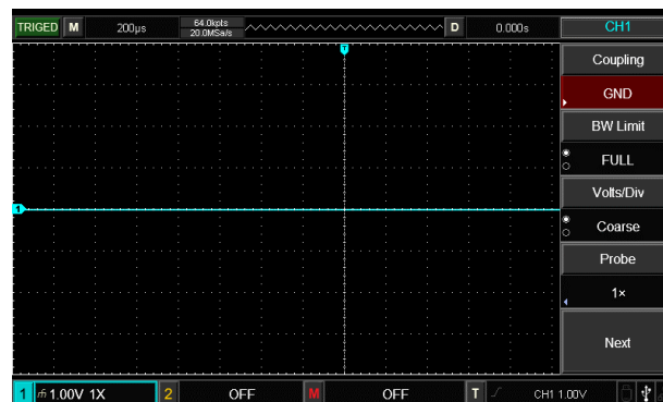
Abbildung 2-3 Gleichzeitige Blockierung von Signal-DC- und AC-Komponenten
