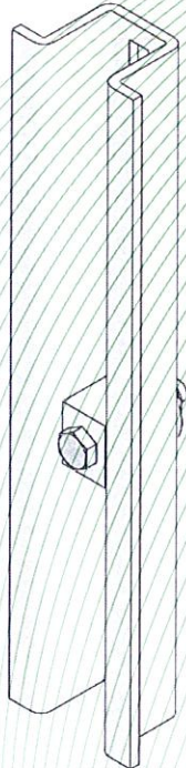
Bild 11: Endsicherung, Schienensperre fest
