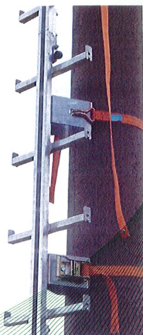
Bild 13: Einholmleiter mit klappbaren Sprossen Bild 14: Einholm-Mastleiter mit Spanngurten
