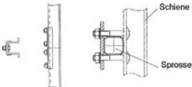
Abb. 1 Verbindung Steigschutzschiene
