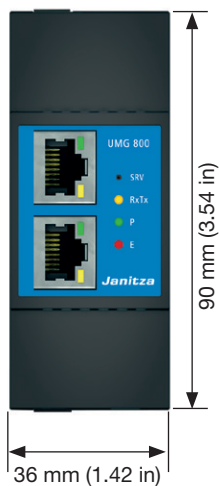
Frontansicht
