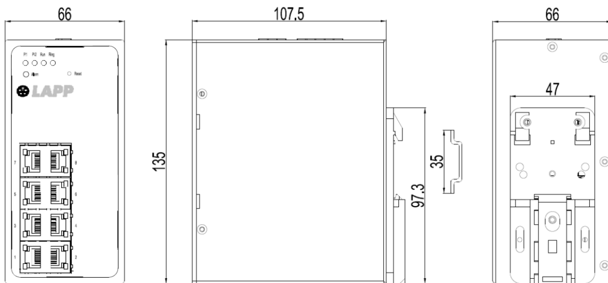
Maßzeichnung (M08T-2GEN)
