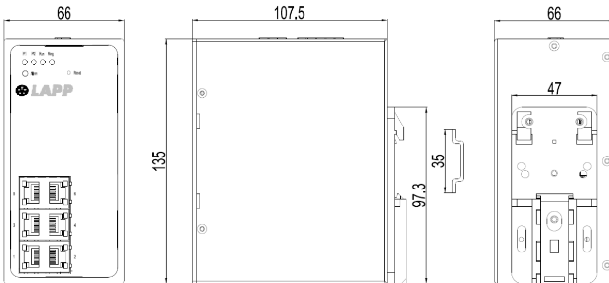
Maßzeichnung (M06T-2GEN)
