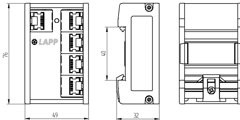
Maßzeichnung (UF05T)
