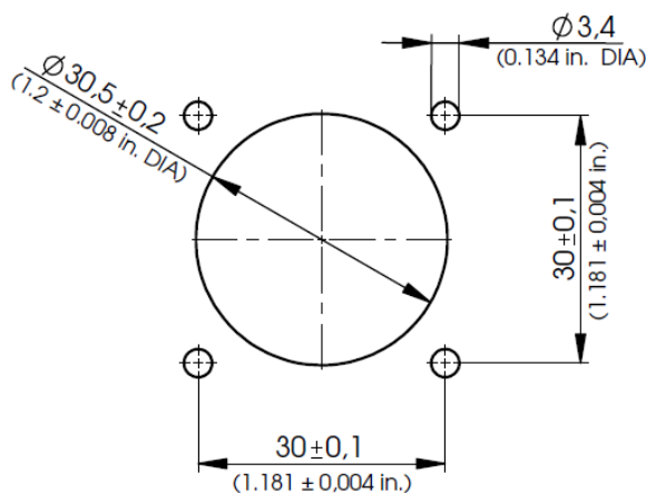
Flansch-Einbaumaße
