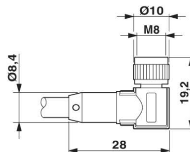
Buchse M8 x 1, gewinkelt, mit LED
