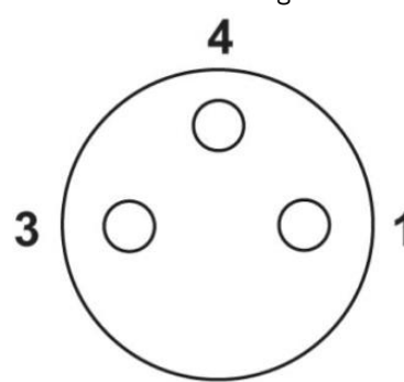
Polbild M8-Buchse, 3-polig, A-kodiert, Ansicht Buchsenseite
