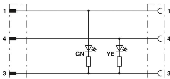
Kontaktbelegung des M8-Stecker und der M8-Buchse, mit LED
