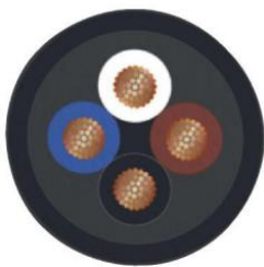
Kabelquerschnitt
