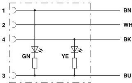
Schaltplan
