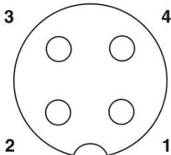
Polbild Buchse M12, 4-polig, A-kodiert, Ansicht Buchsenseite
