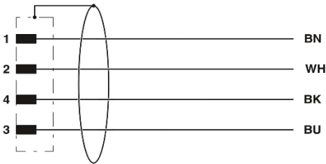
Kontaktbelegung des M12-Steckers
