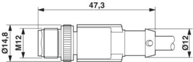
Maßzeichnung
