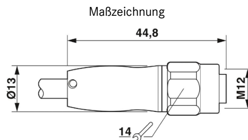
Buchse M12 x 1, gerade
