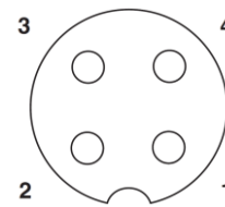
Polbild M12-Buchse, 4-polig, A-kodiert
