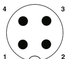
Polbild M12-Stecker, 4-polig, A-kodiert
