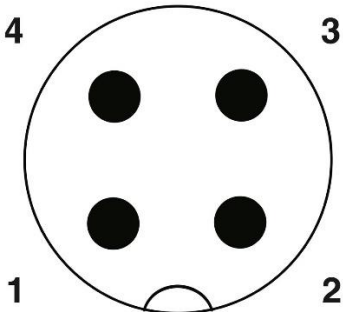
Polbild M12-Stecker, 4-polig, A-kodiert, Ansicht Stiftseite
