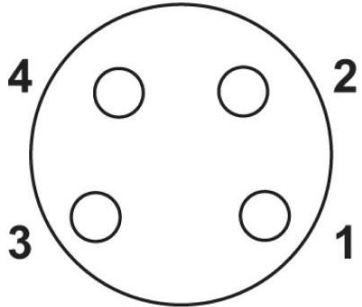
Polbild M8-Buchse, 4-polig, A-kodiert, Ansicht Buchsenseite
